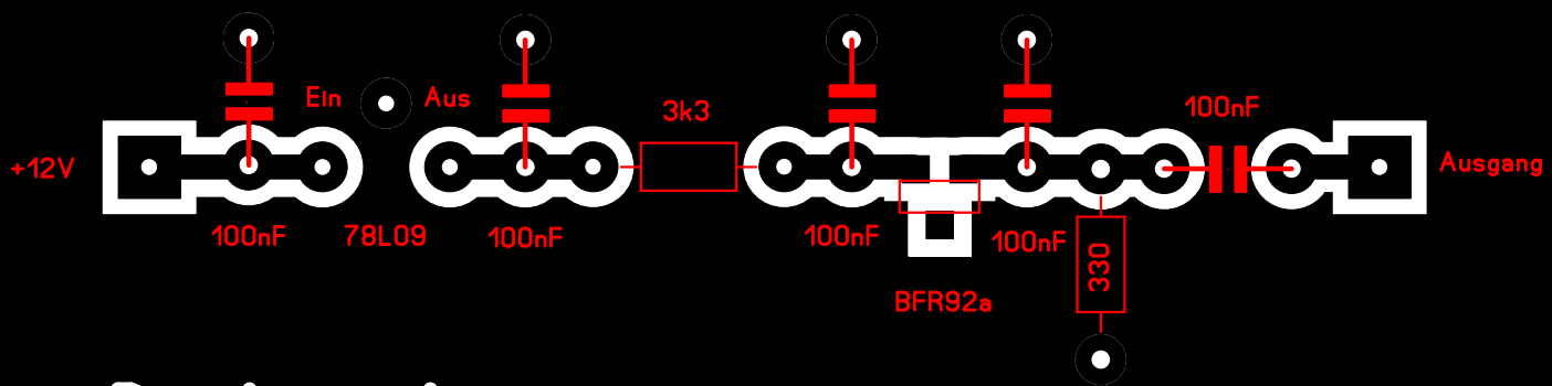
Rauschgenerator
